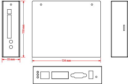
产品外形尺寸图（单位：mm）
